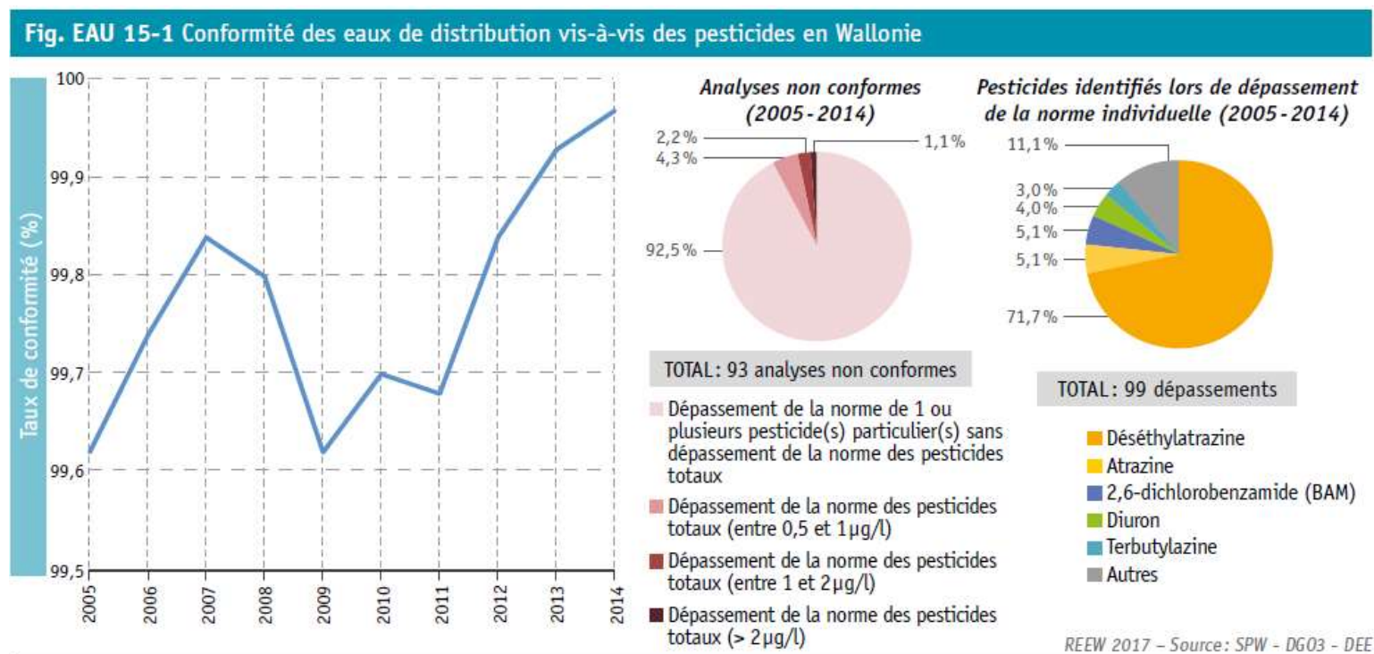
Figure 17 : Taux de conformité des eaux de distribution en Wallonie et paramètres impactants
